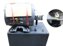
레버식 유압유압모터 / 소음방진 고무결합
